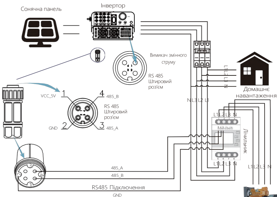
Малюнок 7.4 Схема підключення лічильника Eastron
