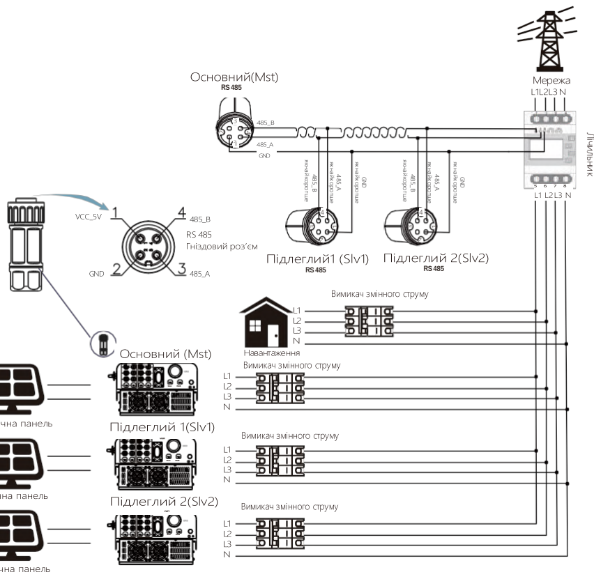
Малюнок 7.19 Схема підключення Eastron (схема прохідних каналів)
