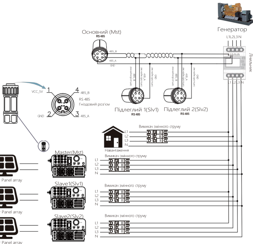
Малюнок 7.21 Схема підключення Eastron (схема проходних каналів)
