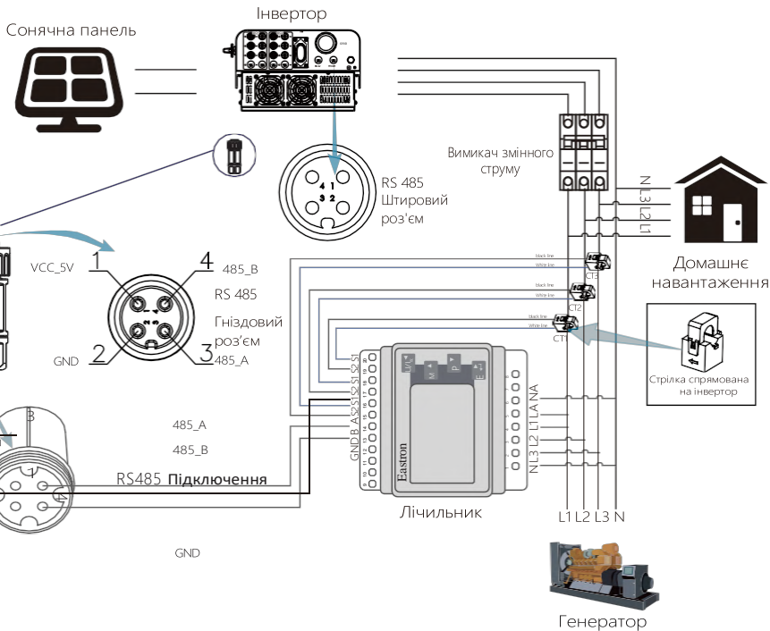
Малюнок 7.8 Схема підключення лічильника Eastron
